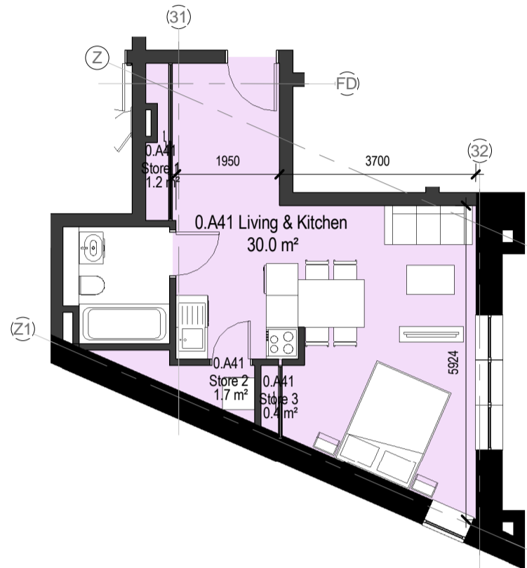
6 Studio Type 0F 1 : 100
