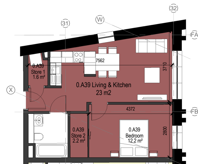
15 1 Bed Type 1F 1 : 100
