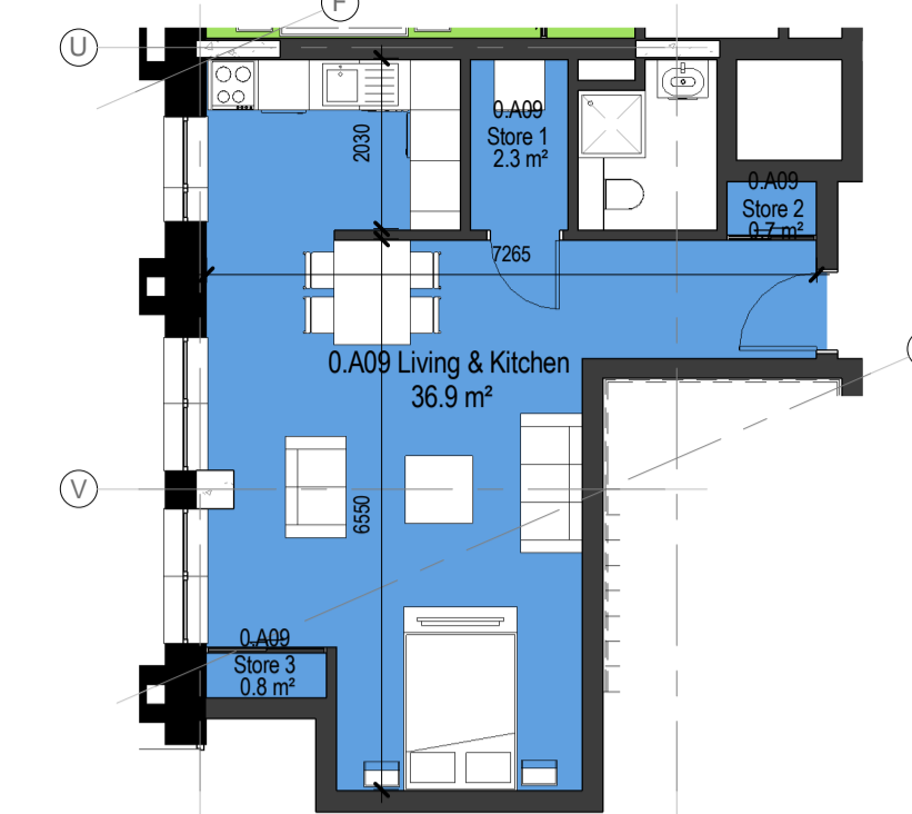
5 Studio Type 0E 1 : 100
