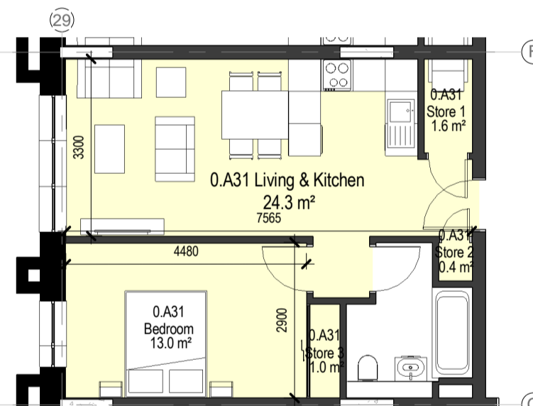
10 1 Bed Type 1A 1 : 100
