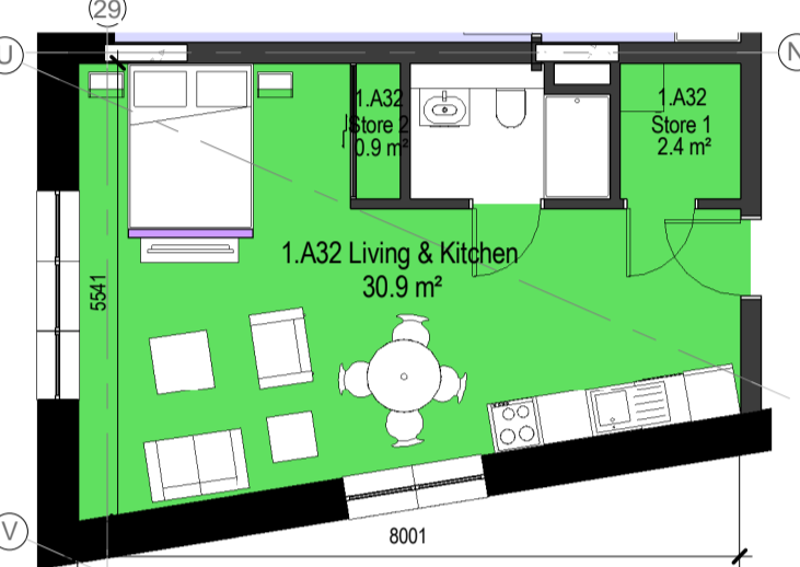
7 Studio Type 0G 1 : 100
